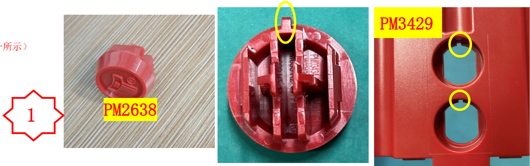
图一，将 2 个 PM2638 凸台对准 PM3429 凹槽，将卡扣扣入孔内，扣合到位（如图一所示）
