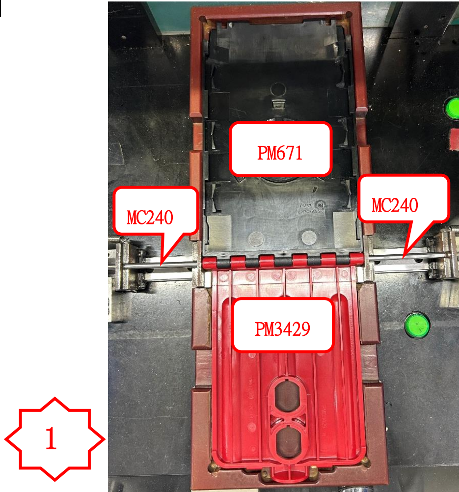
图一, 将 PM3429/PM671 装在治具如图的位置, 再在两边分别放入 MC240 (如图示)
