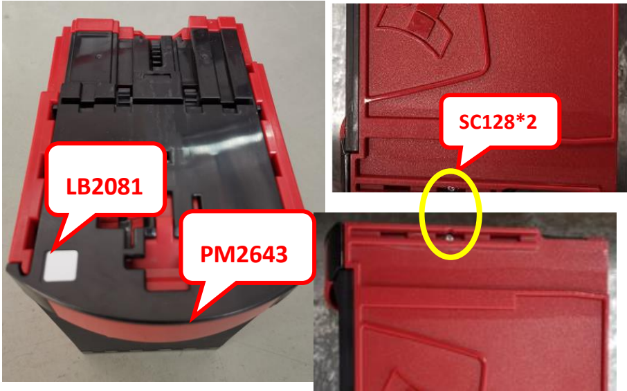
图一，拉动 PM2643,检查是否能回弹顺畅，检查 2 颗 SC128 有无漏打, LB2081 有无漏装
