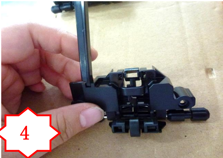
图四,将装好 SP157 的 PM683 装在 PA2742-4 中
