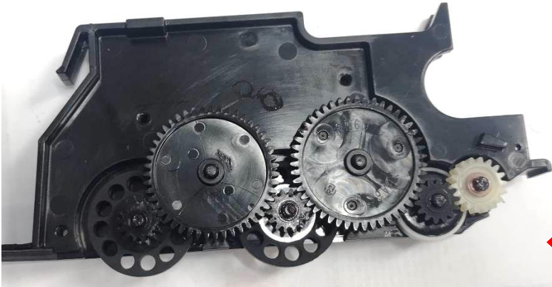
图二，按照图片操作所示，装上 PM697*2。
