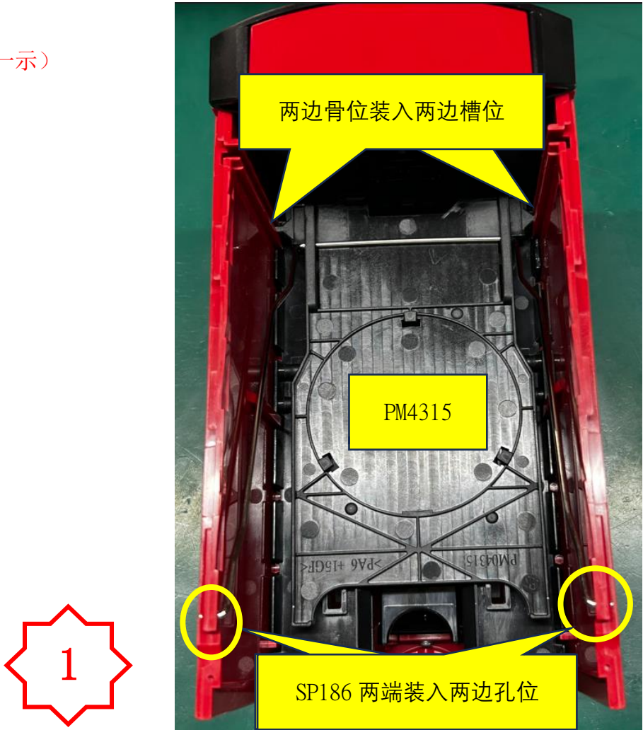
图一，将 PA3845-1 上的 PM4315 两边骨位装入 PM2625 两边槽位，将 SP186 两端插入 PM2625 两侧孔内
