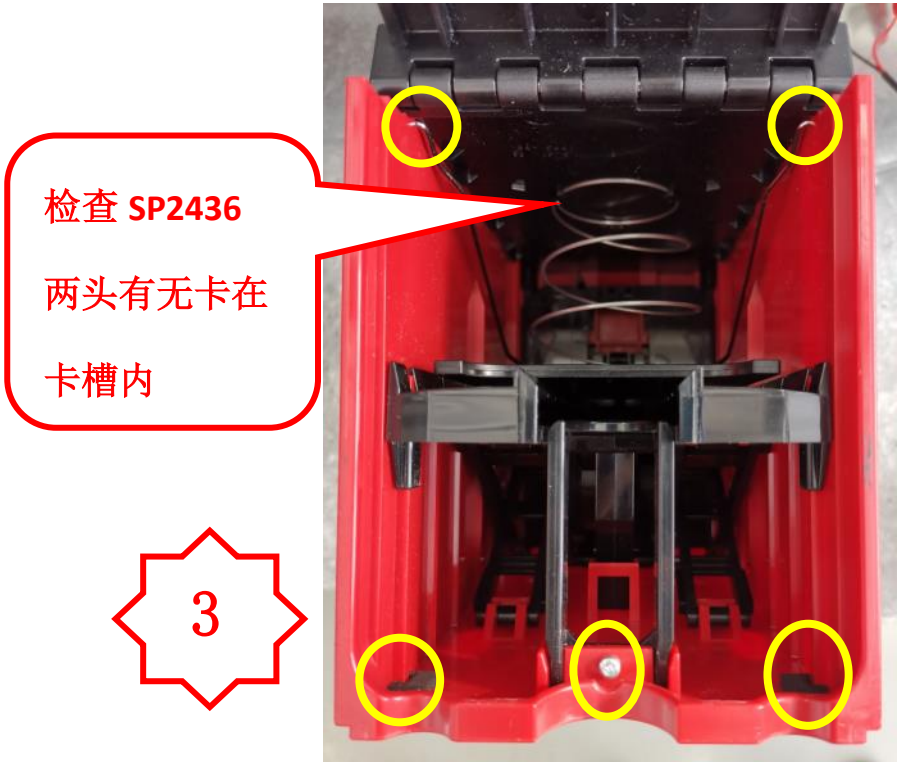
图三，检查 SP186 2 头是否卡在槽中，SP2436 是否卡入槽 内，SC119 有无漏装，4 个 LB2068 有无漏装
