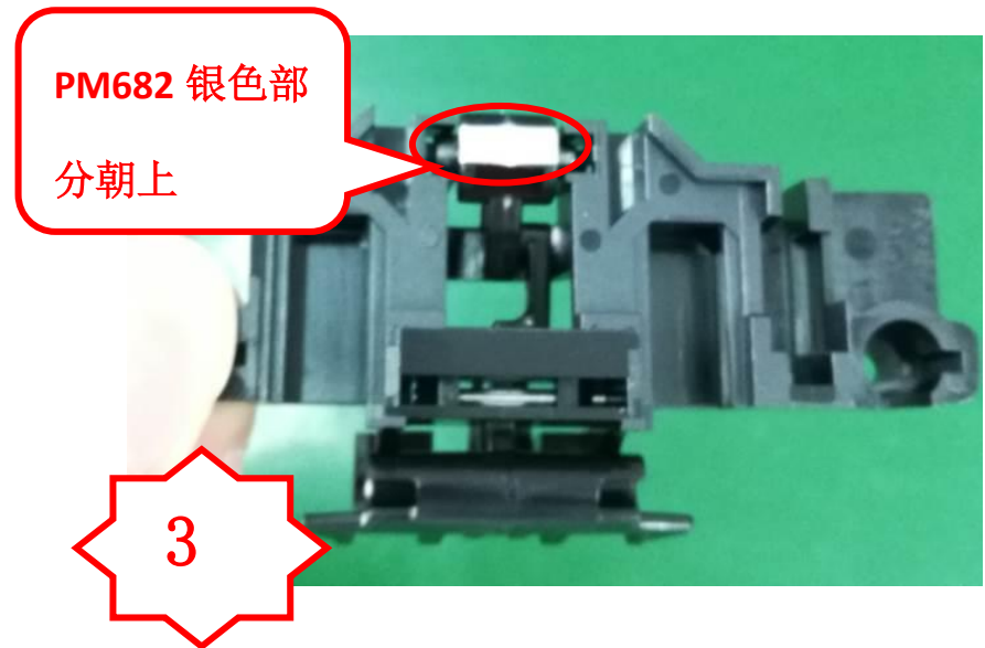
图三, 将 PM682 银色部分朝上装入 PM703, 注意 PM2022 的卡勾要卡在 PM682 的孔内
