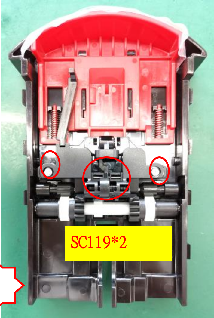
图二，打两颗 SC119，检查 PM654 是否转动顺畅
