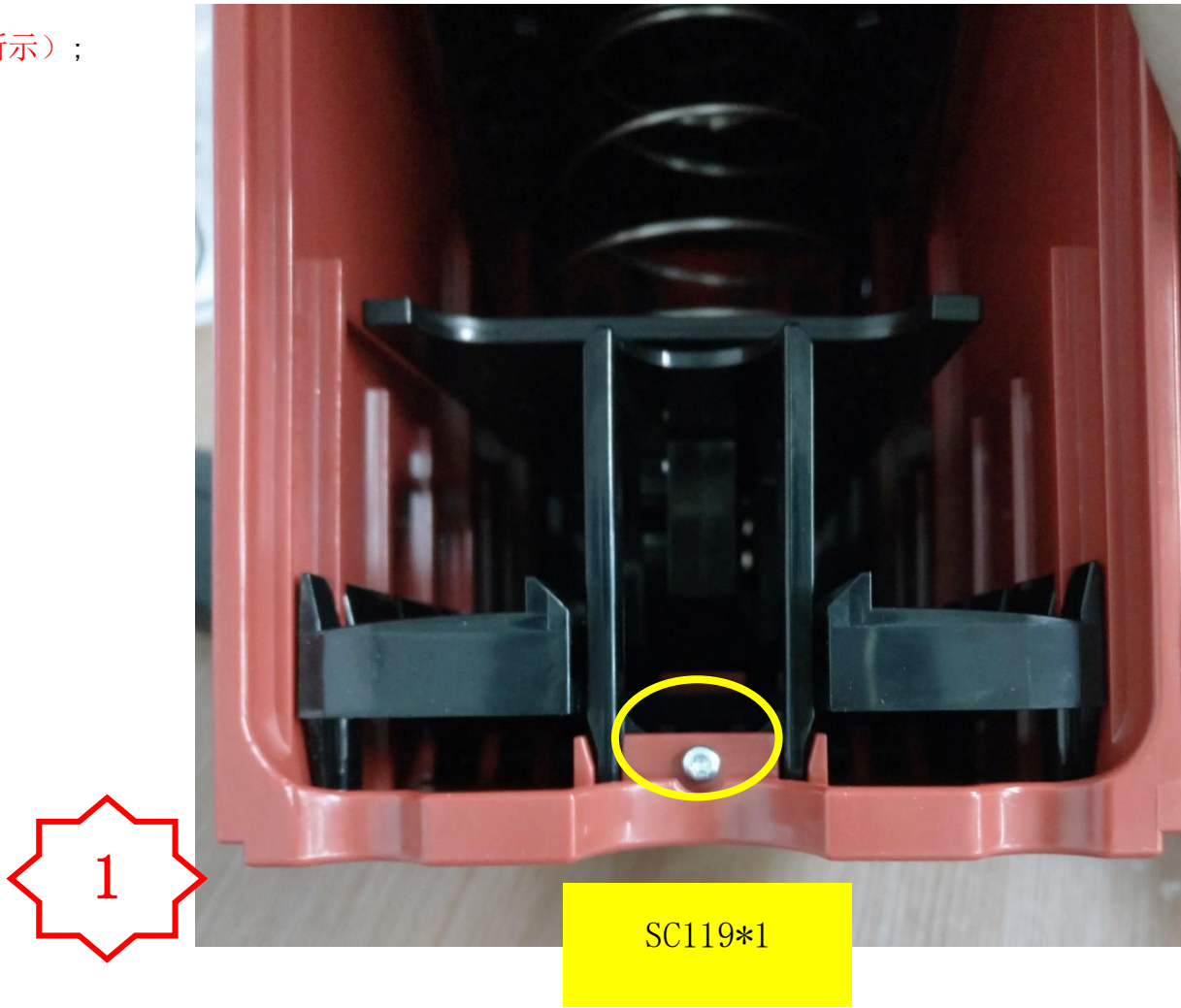
图一，在 PA3845-7 组件上的 PM2625 相应位置中间锁 1 个 SC119 螺丝（如图 1 示）
